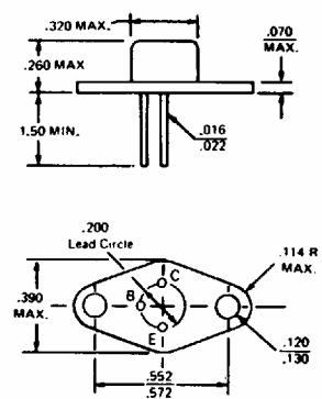
T0-37
