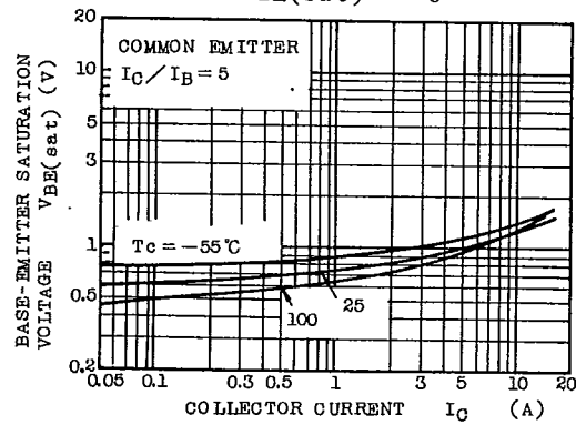
V_{BE(sat)} - I_C
